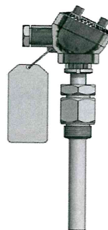
Рисунок 16 - ТП исполнений 113TE03, 114TE03, 215TE10
