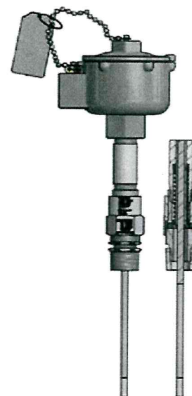
Рисунок 12 - ТП исполнений 111TE10, 112TE09
