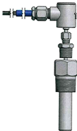
Рисунок 17 - ТП исполнений 113TE03, 114TE03, 215TE10
