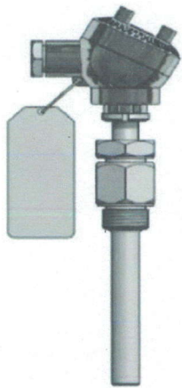
Рисунок 18 – ТП исполнения 215TE11
