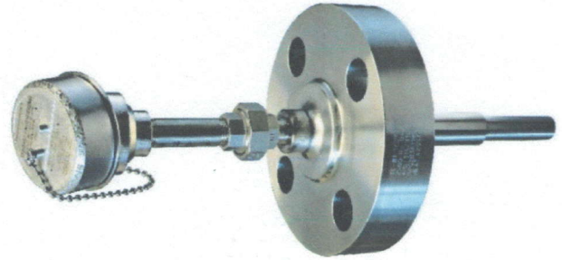
Рисунок 4 – Общий вид ТП исполнений 111TE06, 112TE05, 215TE09
