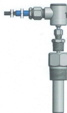
Рисунок 17 – ТП исполнений 113TE03, 114TE03, 215TE10
