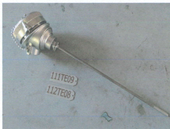
Рисунок 28 – ТП исполнений 111TE09, 112TE08
