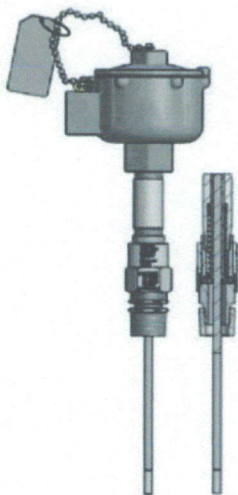
Рисунок 12 – ТП исполнений 111TE10, 112TE09
