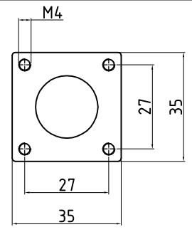
A-A VIEW
